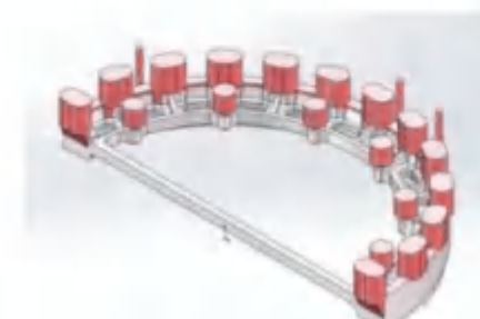
CAE 模拟 CAE simulation
